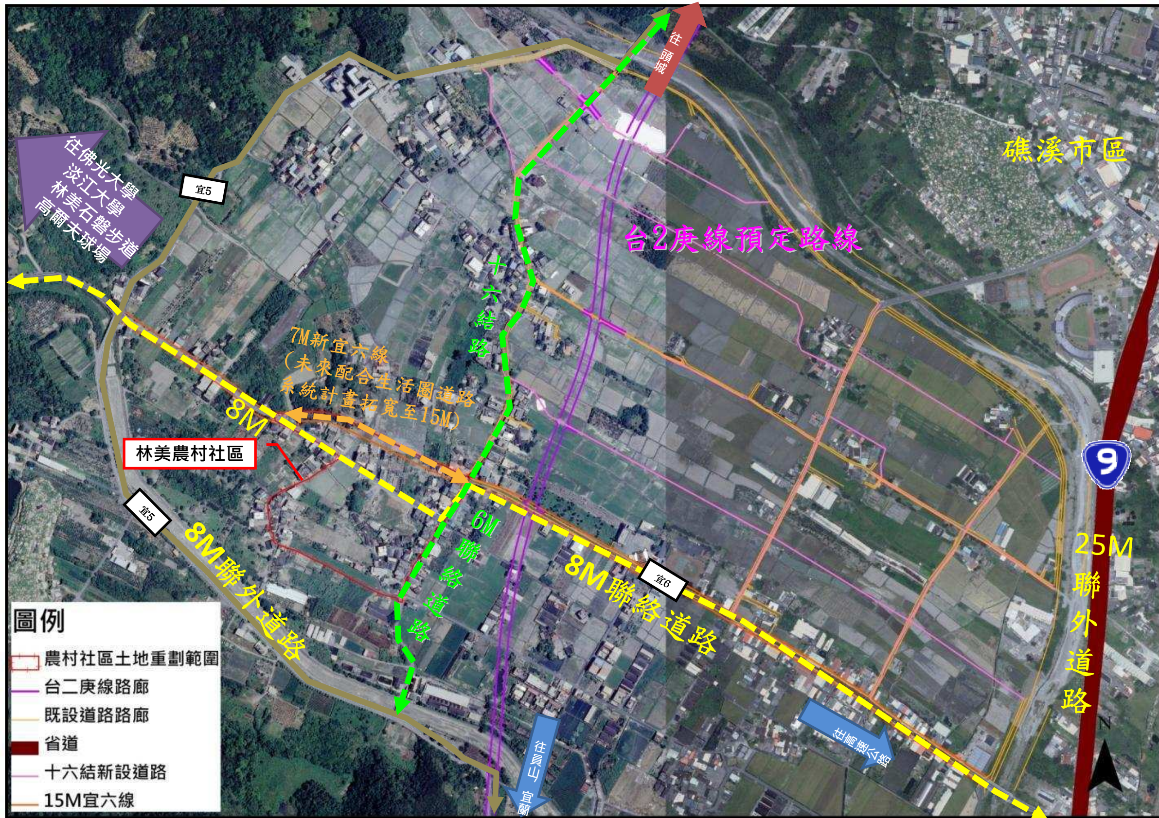
圖 號：3-5 圖 名：聯絡及聯外道路系統圖 申請案名：宜蘭縣礁溪鄉林美農村社區土地重劃非都市土地開發許可作業 申請單位：宜蘭縣政府
